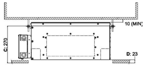
» Abb.9 AQ 10-20-30-35
