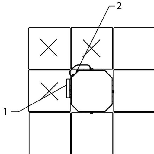
» Installation AQ 40-50-60
