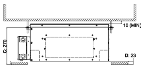
» Fig.9 AQ 10-20-30-35
