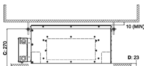
» Fig.9 AQ 10-20-30-35
